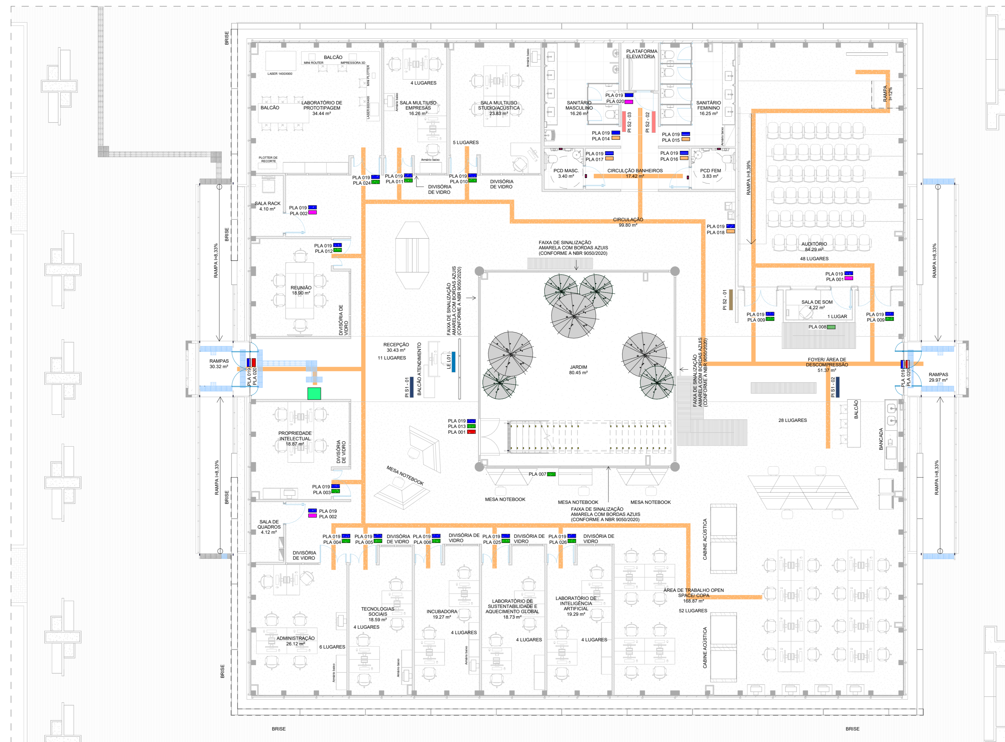
1 PLANTA DE SINALIZAÇÃO E ACESSIBILIDADE - TÉRREO 1 : 100
