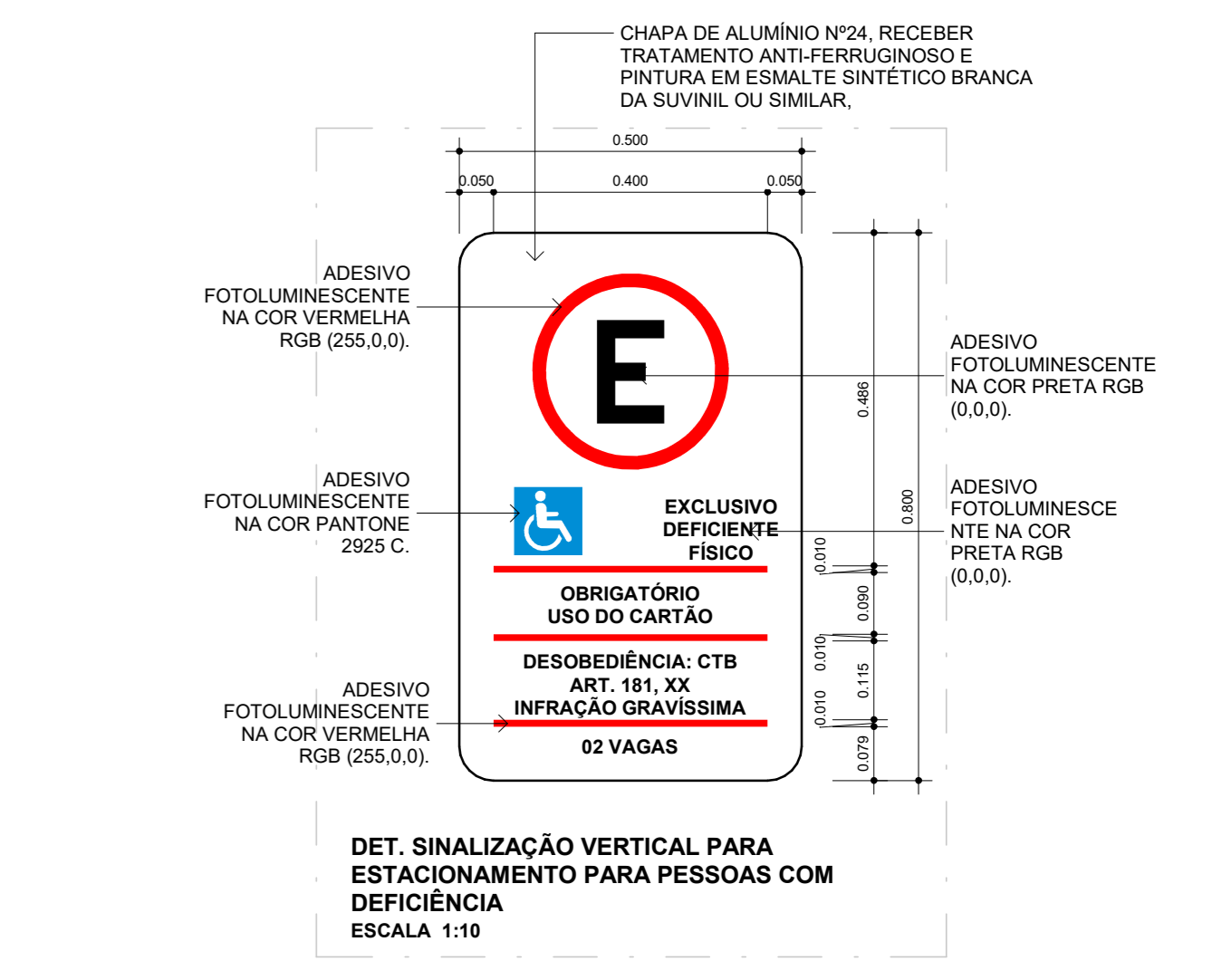
DET. PLACA DE ESTACIONAMENTO 1:10
