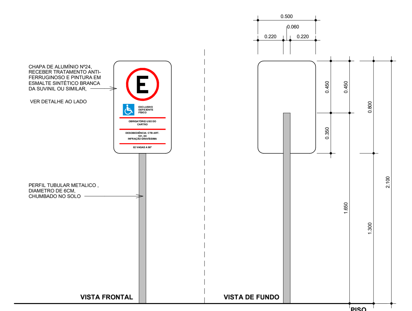
NOVA PLACA DE SINALIZAÇÃO DE VAGA PCD 1:20
