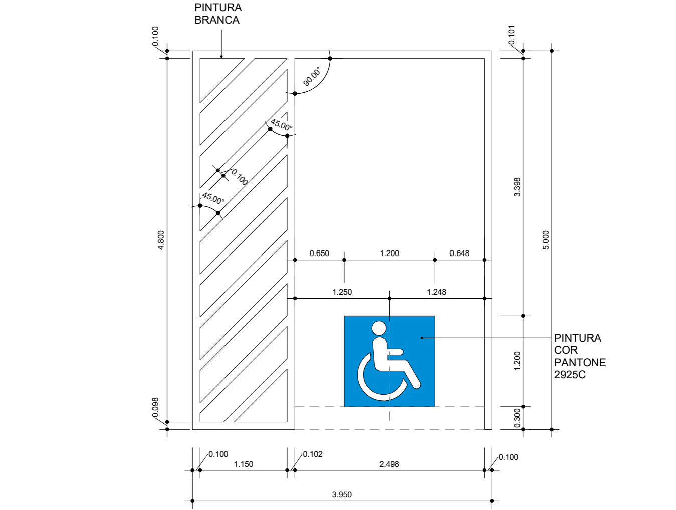
DET. VAGA PCD 1:50
