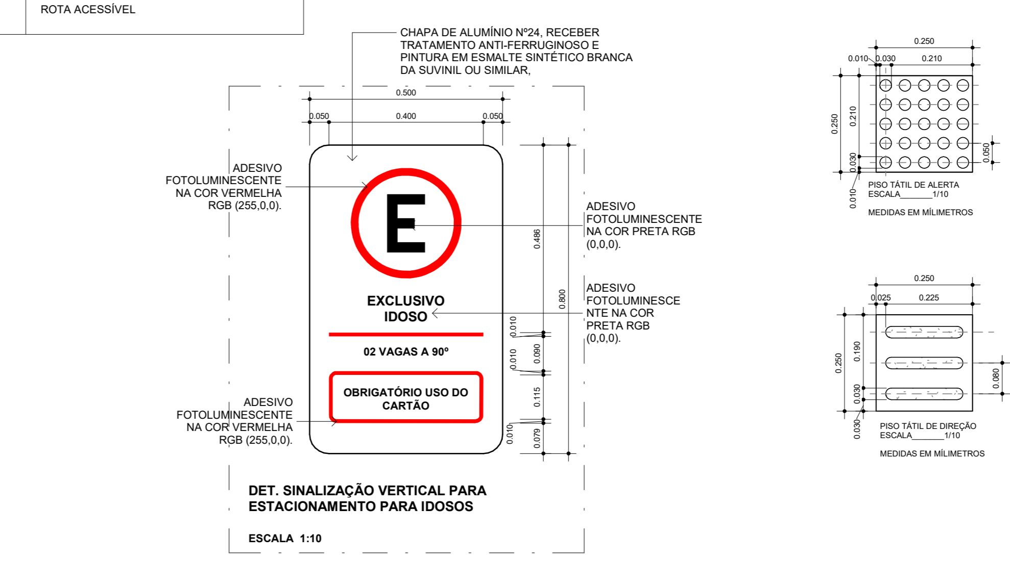
DET. PLACA DE ESTACIONAMENTO IDOSO 1:10
