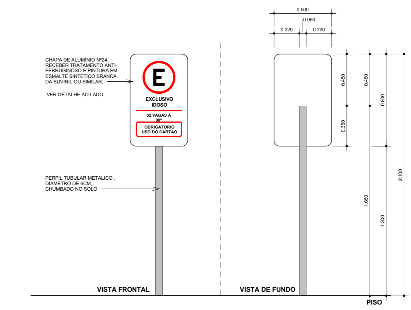
PLACA DE SINALIZAÇÃO DE VAGA IDOSO 1:20
