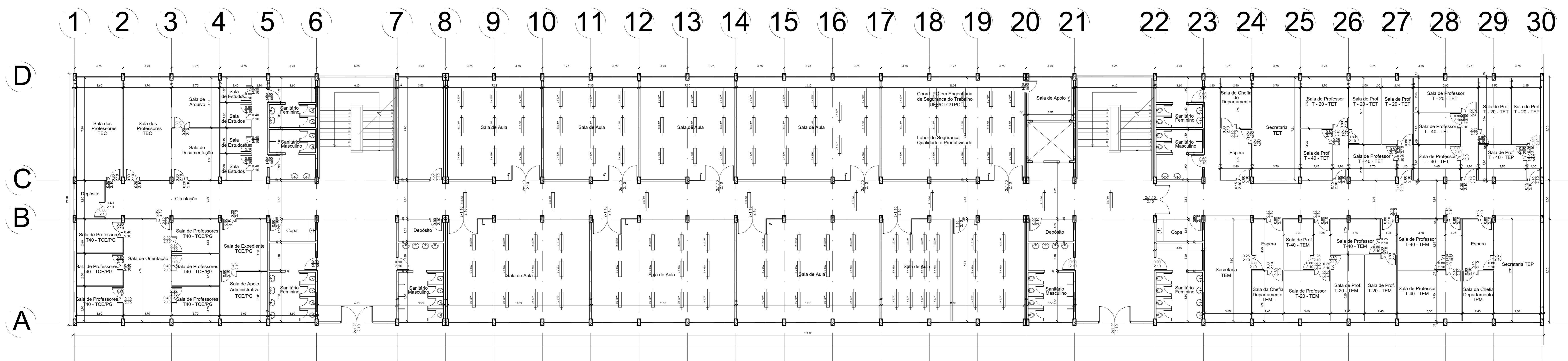
01 PLANTA 4º PAVIMENTO esc. 1/125
