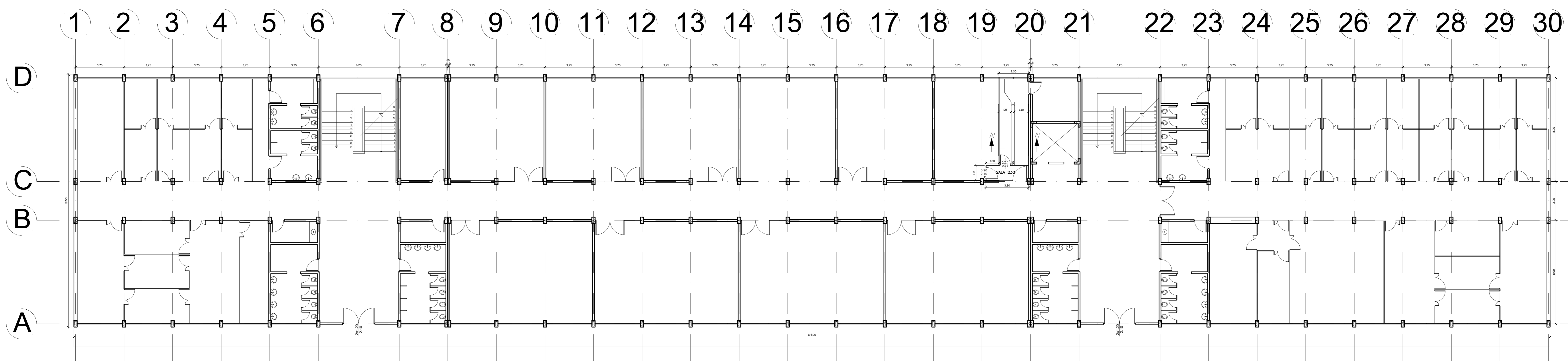
01 PLANTA 2º PAVIMENTO esc. 1/225
