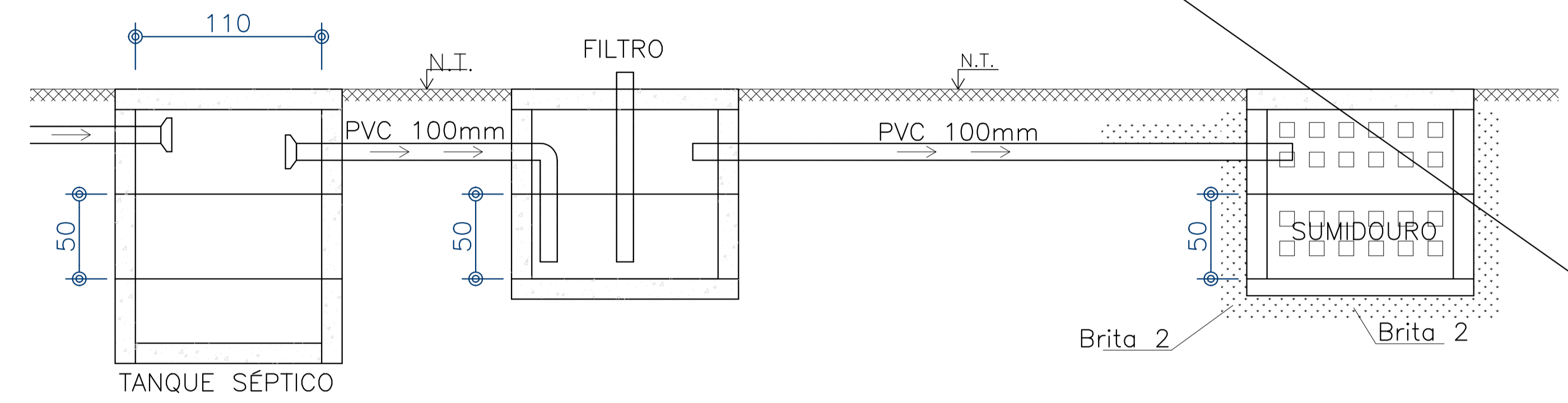
DETALHE DO TANQUE SÉPTICO, FILTRO E SUMIDOURO ESCALA 1/25
