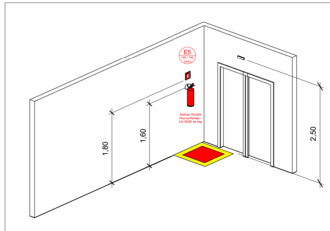
DETALHE FIXAÇÃO DE ELEMENTOS 1:50
