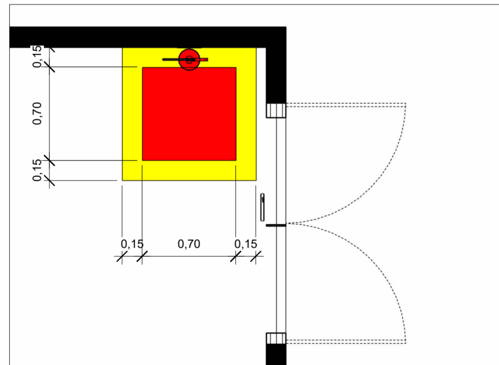
DETALHE SINALIZAÇÃO PISO 1:25
