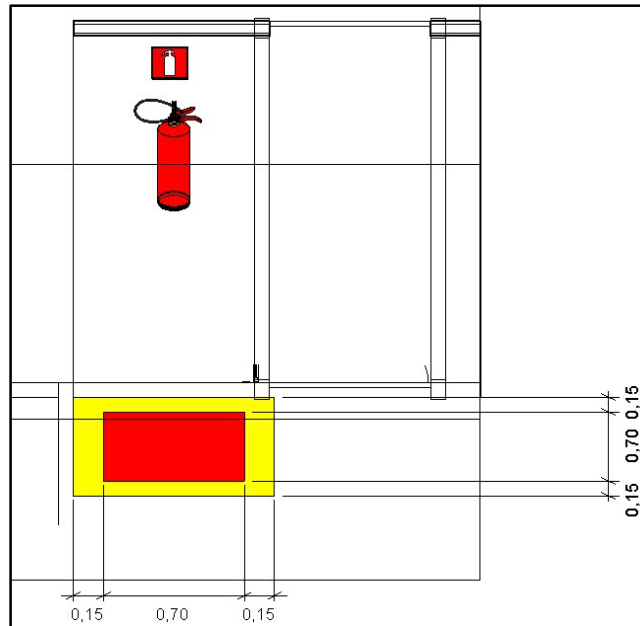
Detalhes da sinalização de extintores no solo
