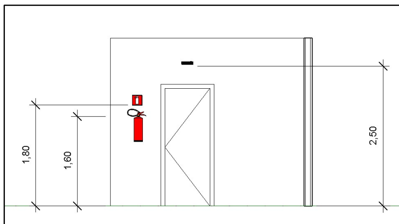
Leiaute Guarita - Extintores, Sinalização de Segurança e Iluminação de Emergência.
