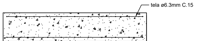
CORTE A-A' ESC.: 1 : 50
