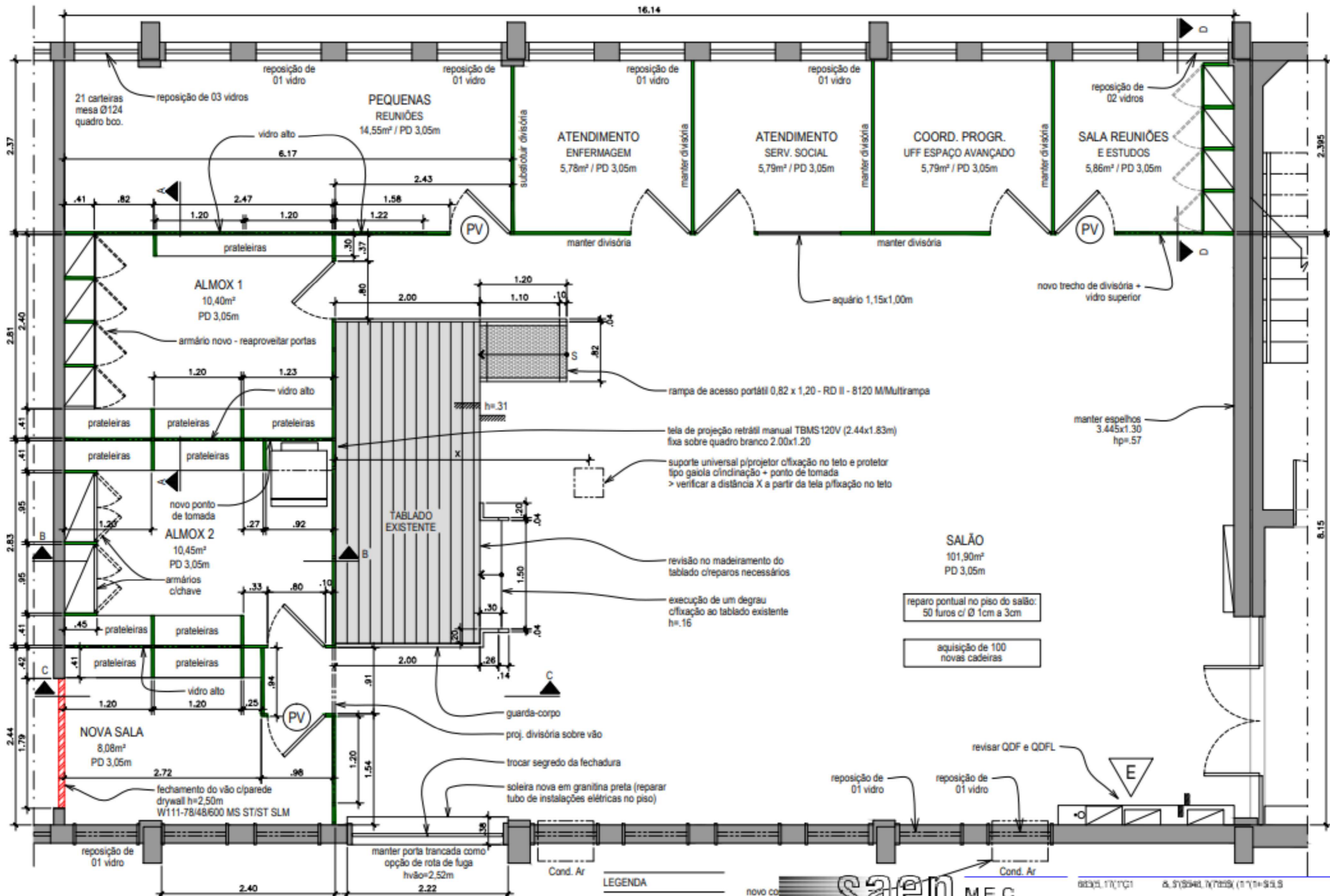
01 PLANTA BAIXA ESCALA: 1/50
