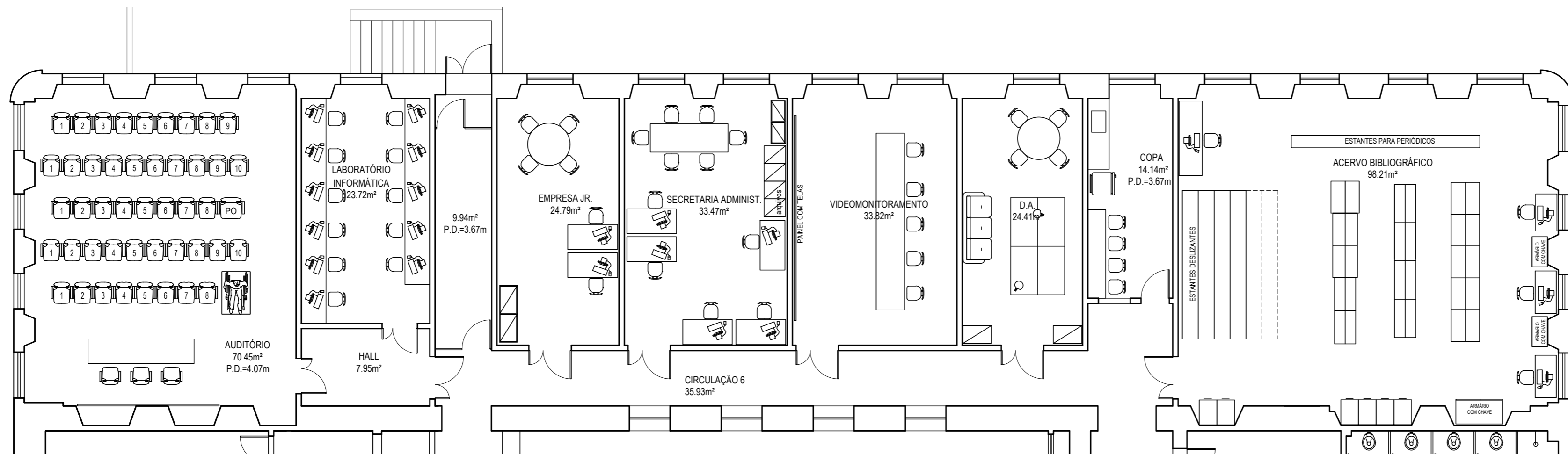
LAYOUT - PAVIMENTO TÉRREO ESCALA 1:100
